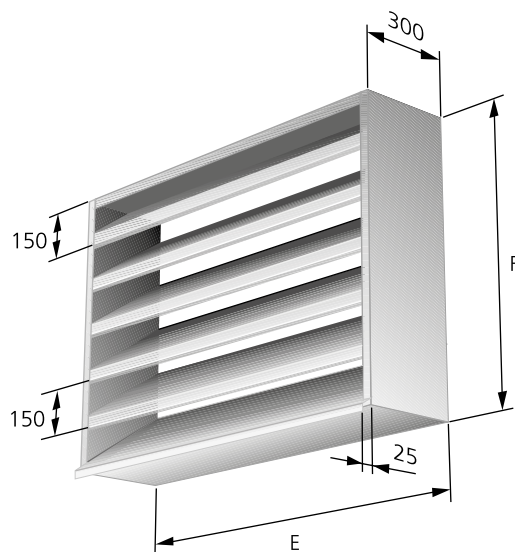
Figur 3. ALD - måttskiss
