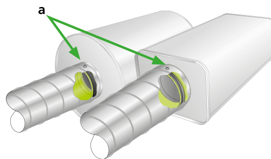
Kuva 1. Paloturvallisuuden vuoksi kanavat kiinnitetään liittimen sisään valettuun peltireunaan ruuvilla tai popniitillä (a).
