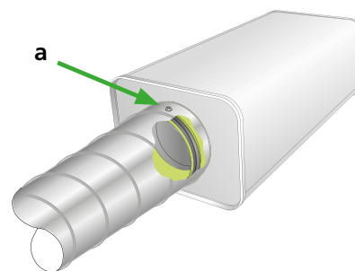
Figur 1. För brandsäkerhets skull, fästs anslutningskanalen i den uppdragna plåtkanten som är fastgjuten inuti anslutningstosen med skruv eller popnit (a).
