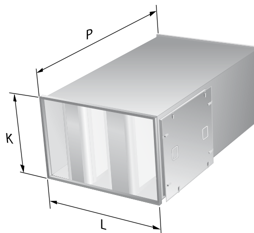
Kuva 5. mittapiirustus
